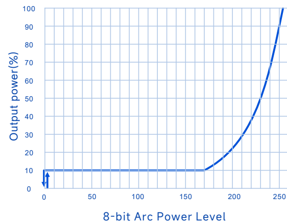
对数调光曲线:(DALI-2/DMX机型)
