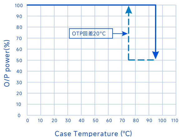
输出功率Vs.壳温(D机型)
